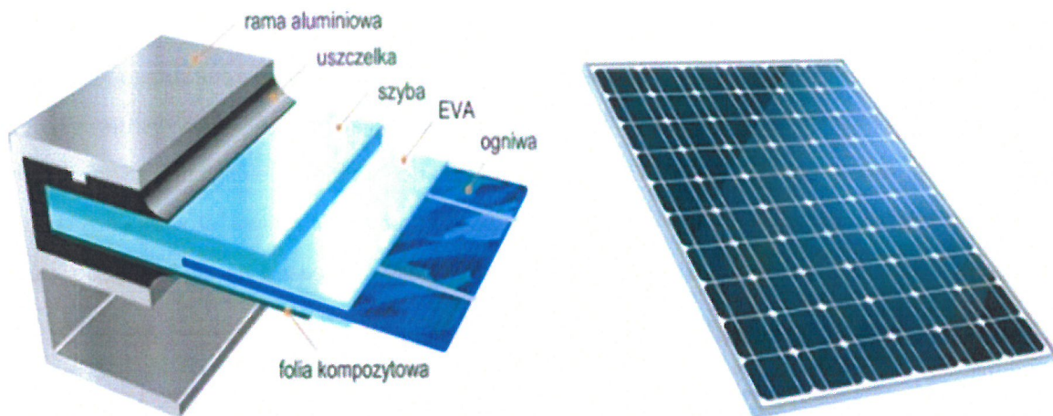
Ryc. Nr 7 Budowa modułu fotowoltaicznego
