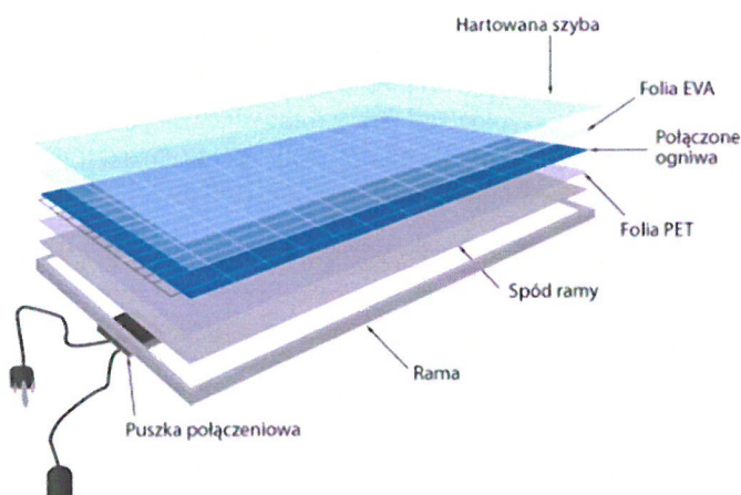
Rys. 3.2. Budowa panelu fotowoltaicznego
