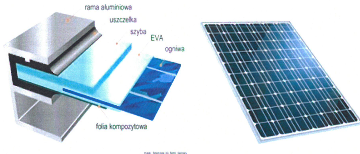
Ryc. nr 7 Budowa modułu fotowoltaicznego
