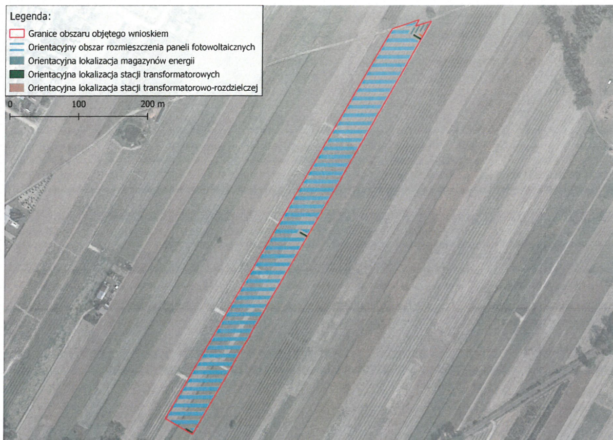
Ryc. nr 13 Orientacyjne rozmieszczenie elementów farmy fotowoltaicznej, ostateczne rozmieszczenie elementów zostanie zaplanowane w ramach projektu budowlanego. (Na podstawie Ortofotomapa GUGiK)
